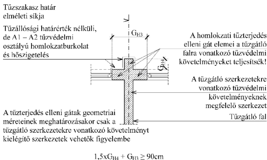
Vízszintes homlokzati tűzterjedés elleni gát metszete
