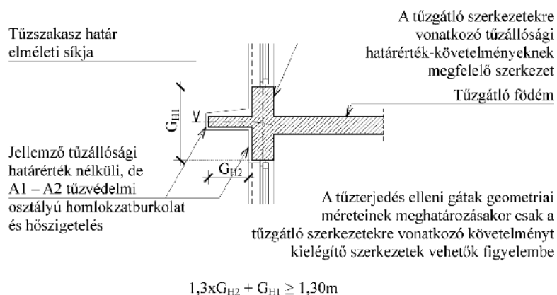
Függőleges homlokzati tűzterjedés elleni gát metszete
