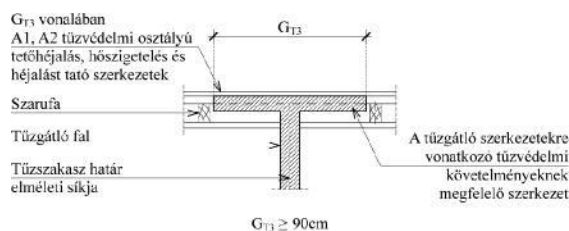
Magastető tetősíkban tartott tűzterjedés elleni gátjának metszete
